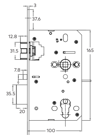
Merlion 鎖匣圖
