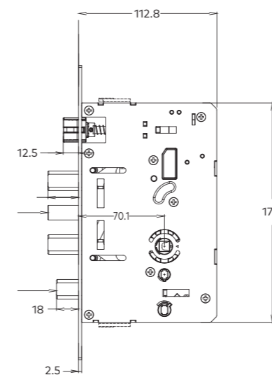
FSL800 鎖匣圖
